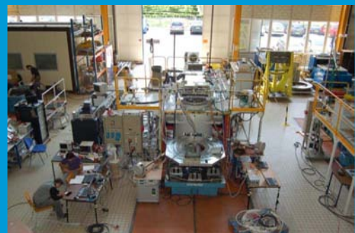
Hall dédié aux essais de vibrations électrodynamiques Hall dedicated to electrodynamic vibrations tests
